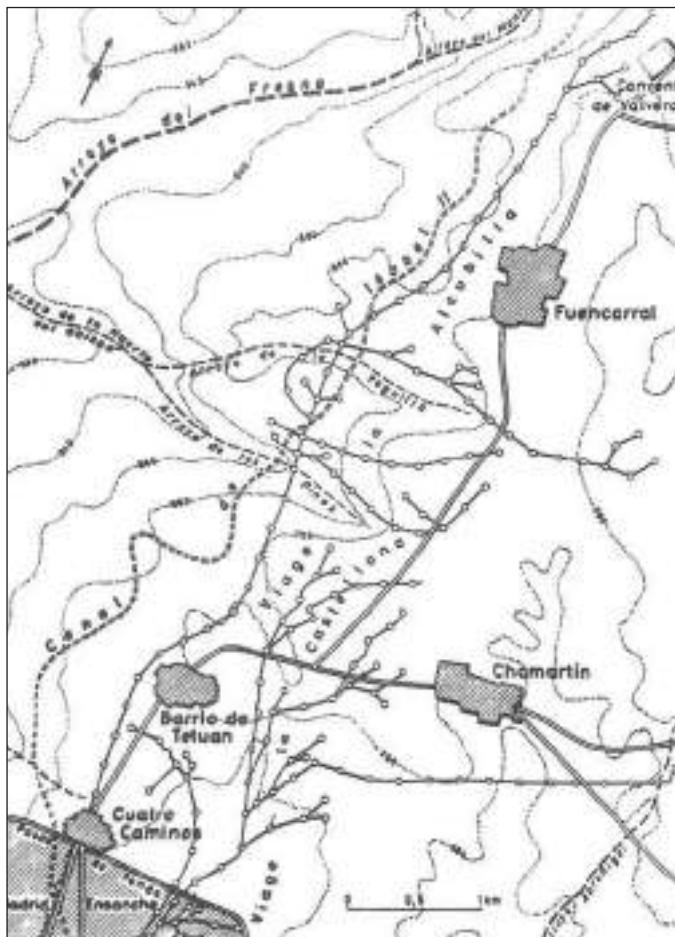
Trazado de los viajes de la Alcubilla y de la Castellana, desde su origen hasta la ronda del Ensanche, según plano de Núñez Granés de 1910.
