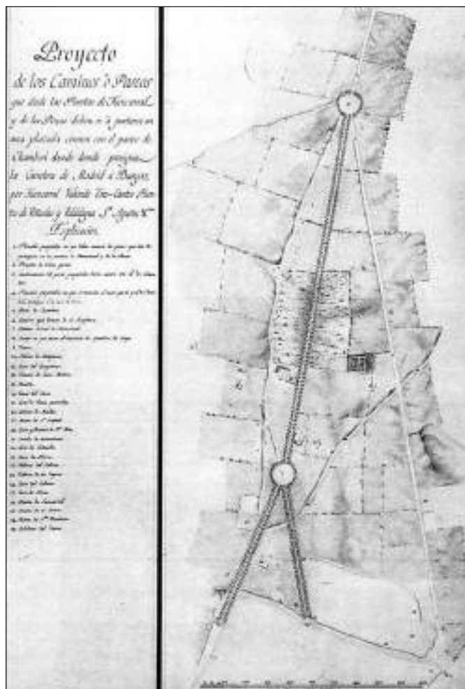
Proyecto de los Caminos o Paseos que desde las Puertas de Fuencarral y de los Pozos deben ir a juntarse en una plazuela común con el paseo de Chamberí desde donde prosigue la Carretera de Madrid a Burgos, por Fuencarral, Valverde, Tres Cantos, Puentes de Viñuelas y Valdelagua, San Agustín, hacia 1800.
